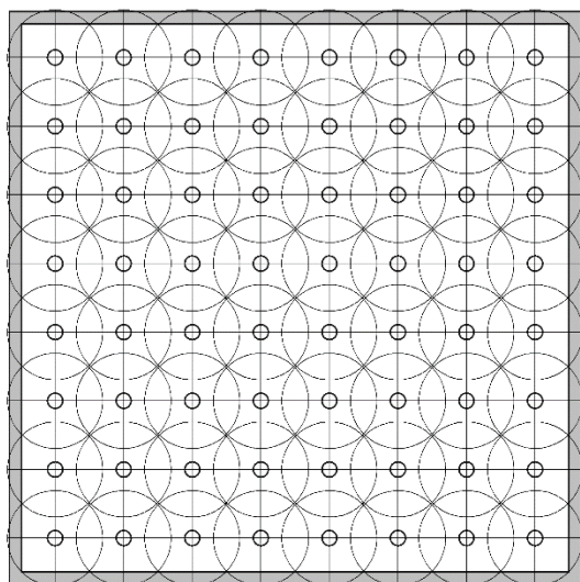
квадратный порядок
